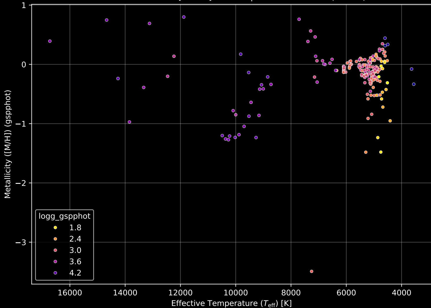
APOGEE DR17 Field: [206-04] Stellar Population Parameters (n= 208)
